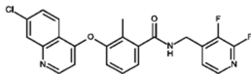
Formula (CXCI)
