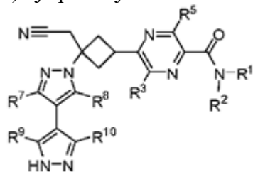
IVa
