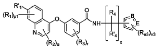
Formula (VIIa-a)
