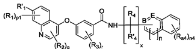
Formula (VIIIa-a)
